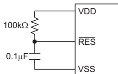
基本复位电路
