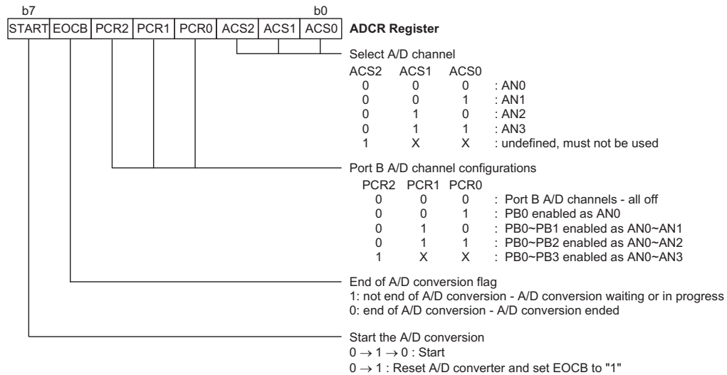
A/D 转换控制寄存器
