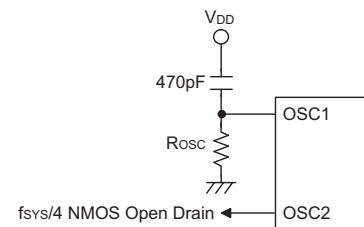
RC 振荡器
